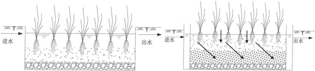
图 4-11 表面流式人工湿地图（b）水平潜流式人工湿地
