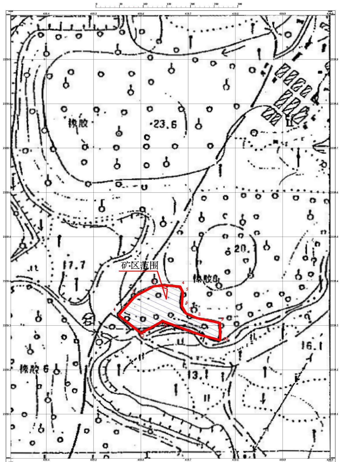
麻章区湖光农场四队那郁河玄武岩矿区地形图
